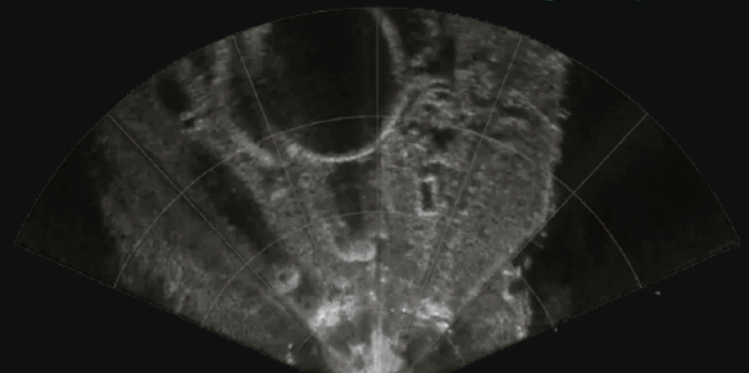
ROV onderwaterscan
